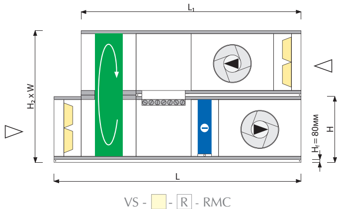
Типоразмеры VS 21÷650
